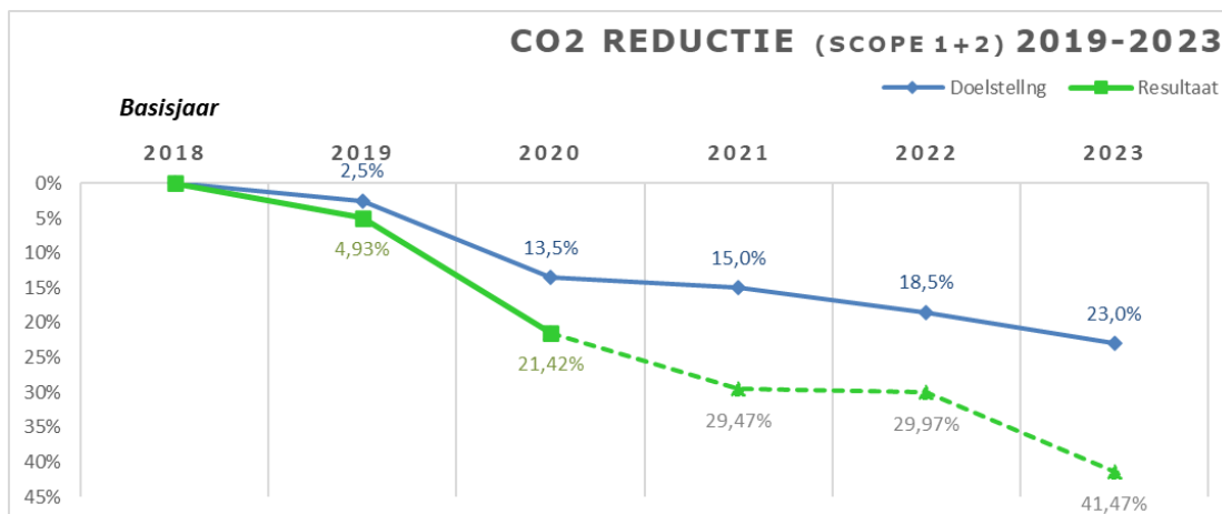
Figuur 8.5.1: Trend en Voortgang reductie doelstellingen (Bron: Footprint CO 2 Roelofs).
